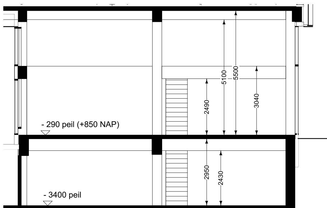
Doorsnede AA'(schaal 1:100)
