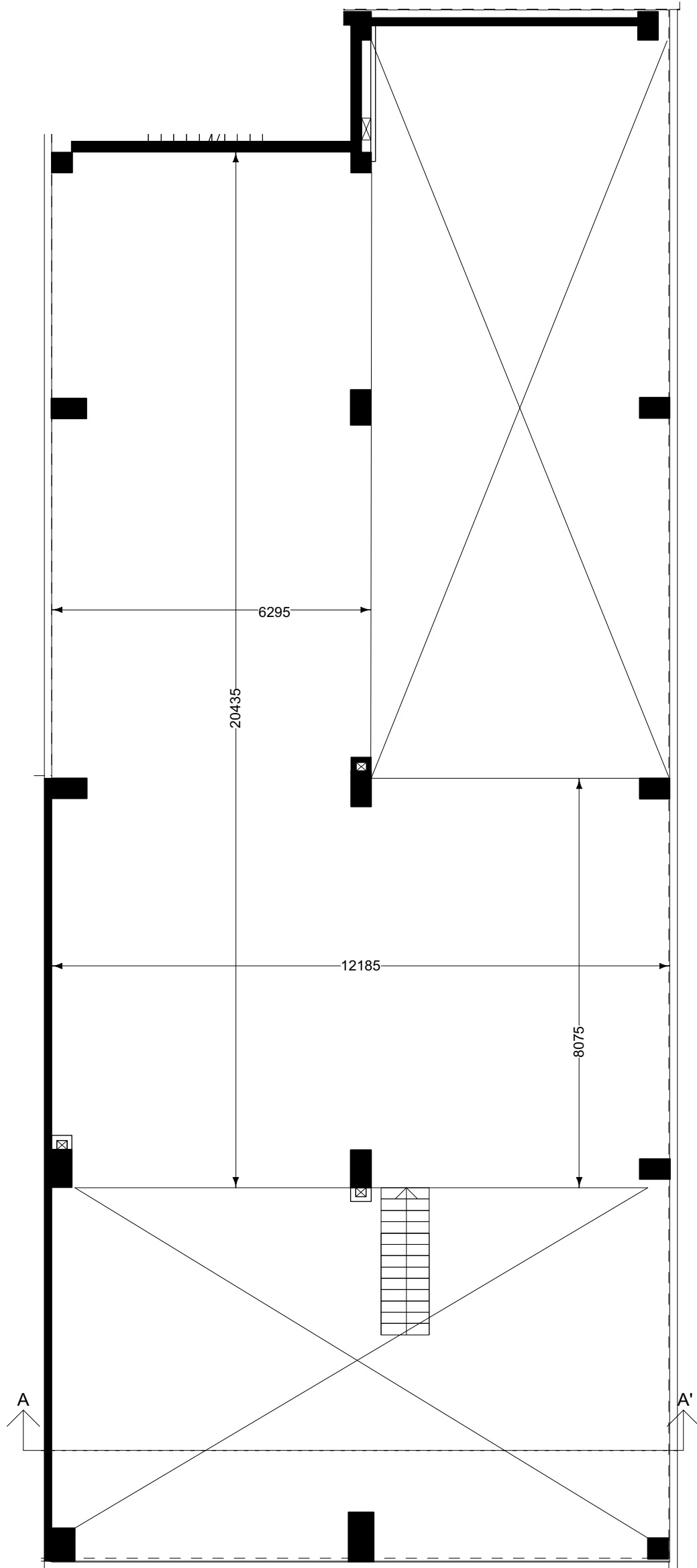
Tussenverdieping (schaal 1:100)
