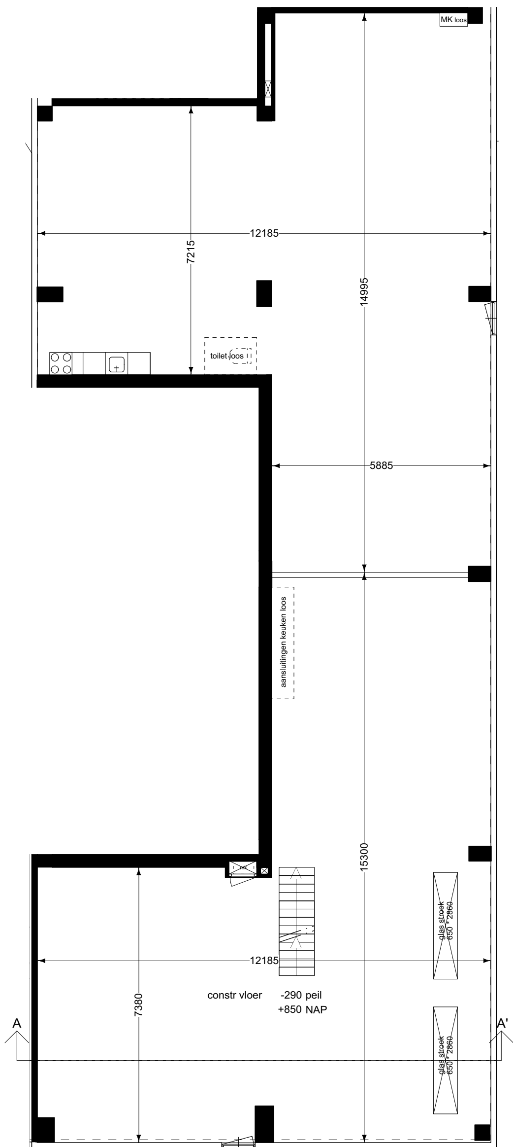
Begane grond (schaal 1:100)
