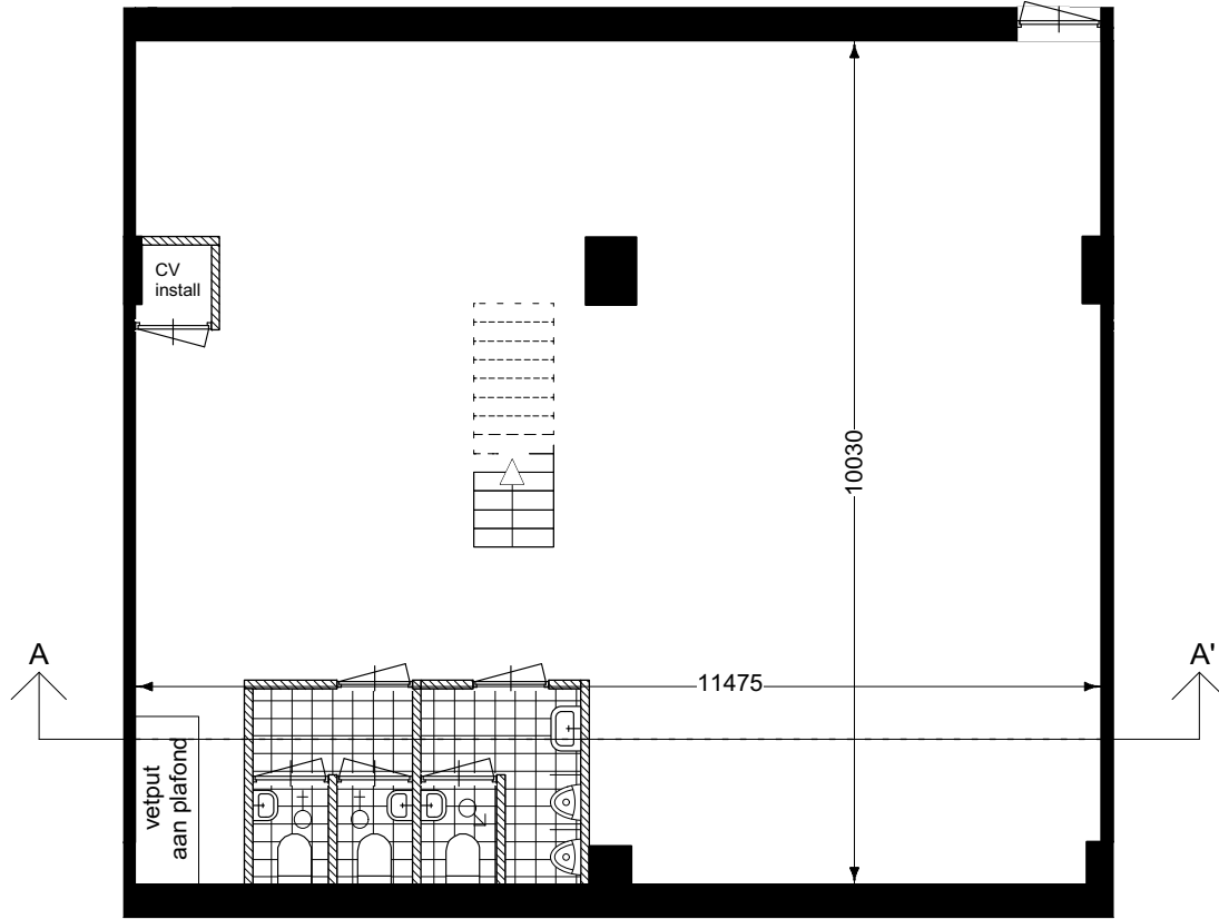
Kelder (schaal 1:100)
