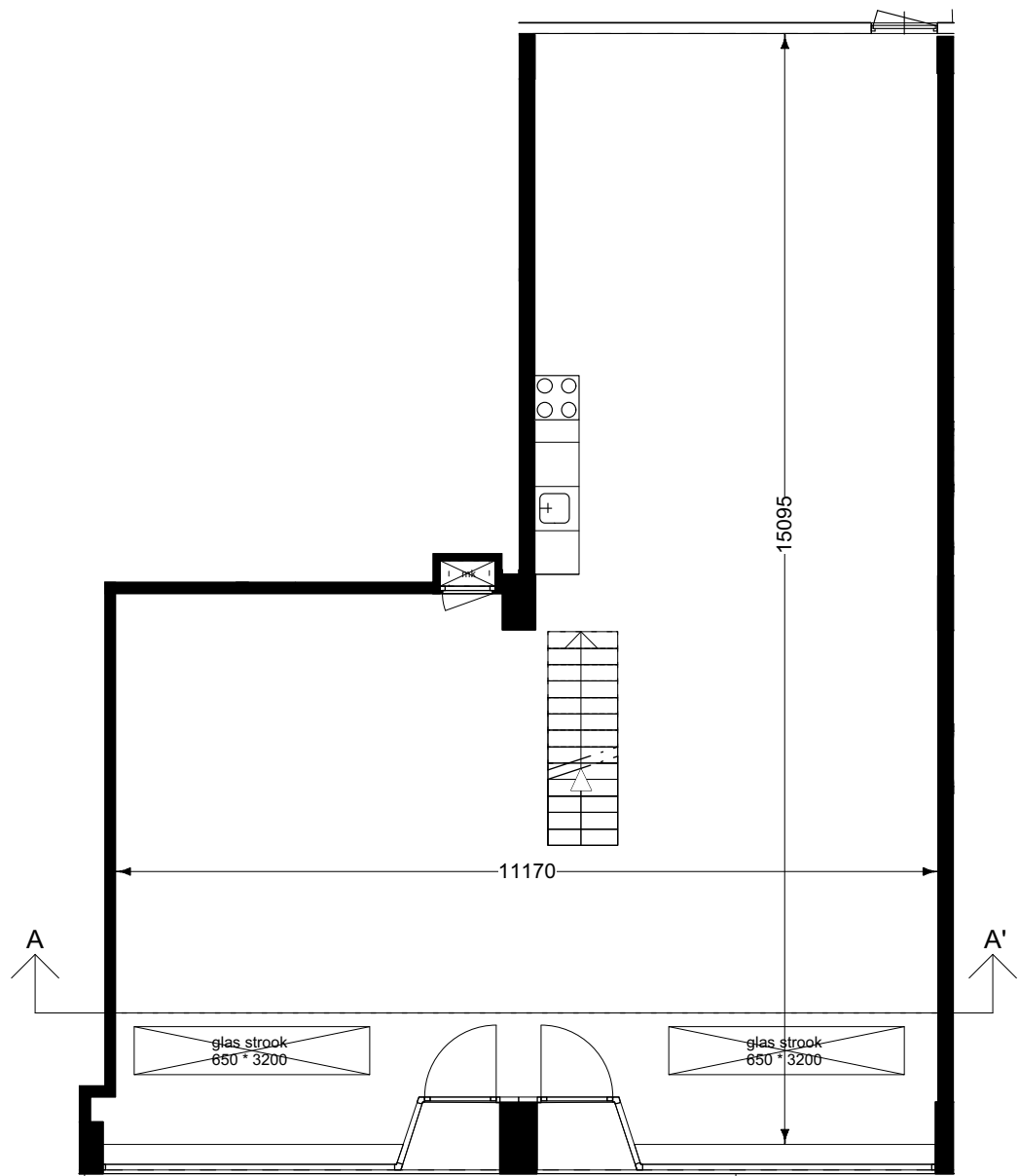
Begane grond (schaal 1:100)
