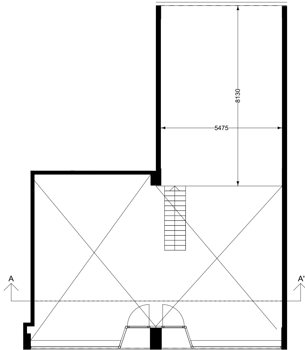
Tussenverdieping (schaal 1:100)
