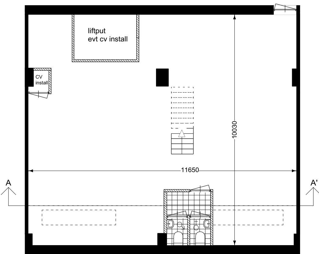
Kelder (schaal 1:100)
