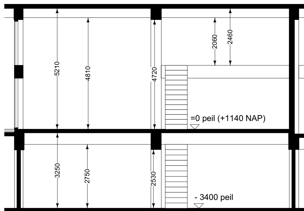
Doorsnede AA'(schaal 1:100)
