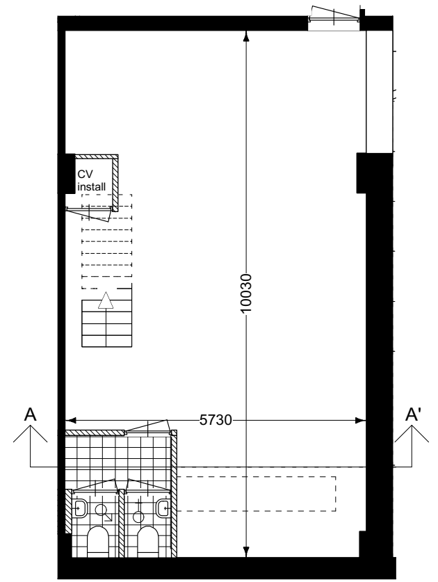
Kelder (schaal 1:100)
