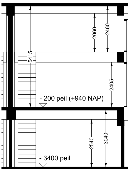
Doorsnede AA'(schaal 1:100)
