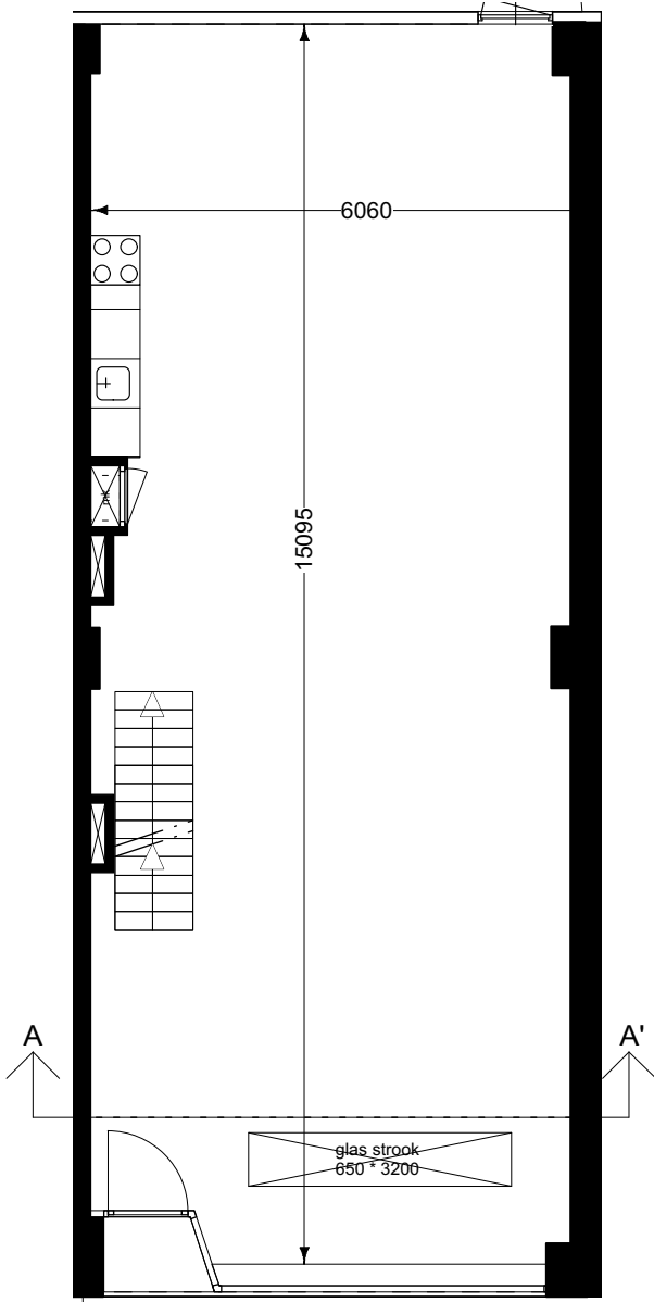
Begane grond (schaal 1:100)
