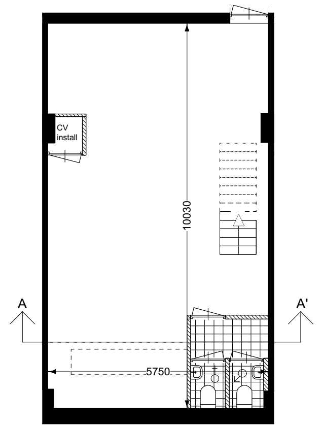
Kelder (schaal 1:100)
