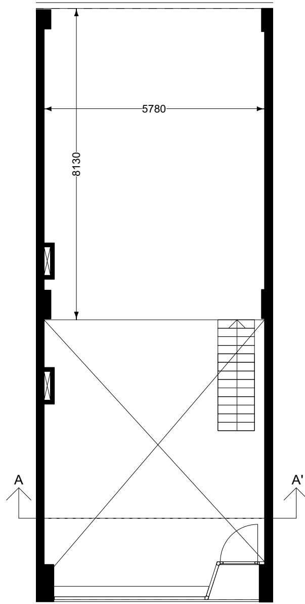
Tussenverdieping (schaal 1:100)
