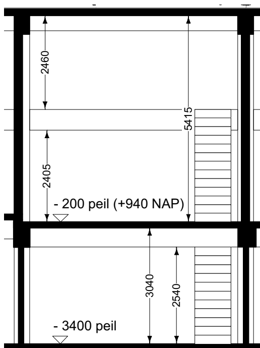
Doorsnede AA'(schaal 1:100)
